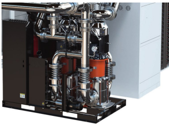
撬装泵组: 冗余泵、过滤与阀组 (渲染图)
