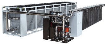
与集成干冷器配套的一次侧回路
